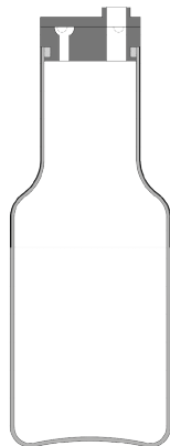
Corte 1-1' esc:1/2
