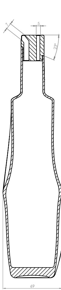
SECÇÃO B-B
