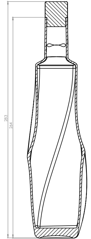
SECÇÃO A-A
